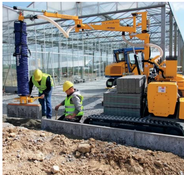
TRANSMOBIL TM elhelyező hordozó a szegélykövek beépítéséhez
