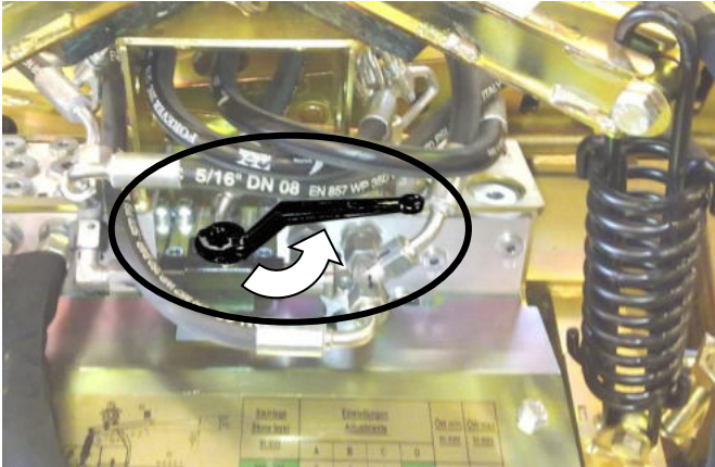
Geöffneter Abstellhahn (Durchflussrichtung) → Nebenspannung in Betrieb
