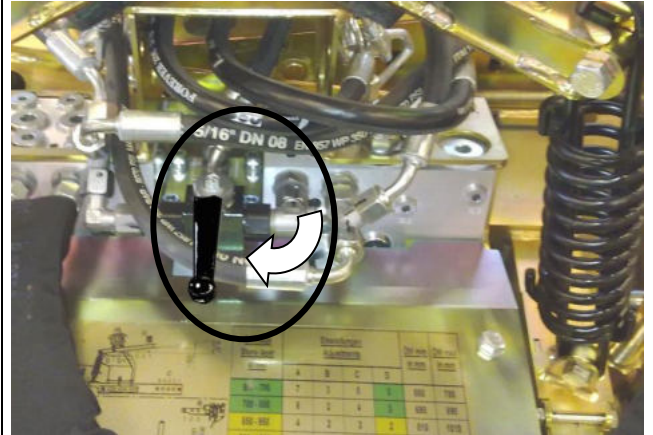
Geschlossener Abstellhahn (Sperrstellung) → Nebenspannung außer Betrieb
