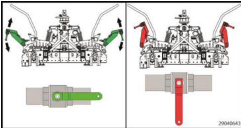
Aufkleber für Sperrstellung der Seitenspannung
